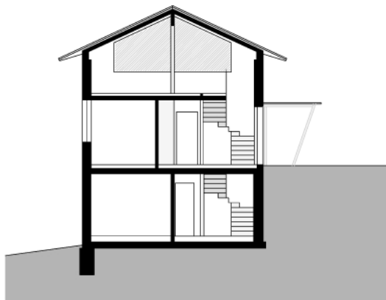
SCHNITT A-A
